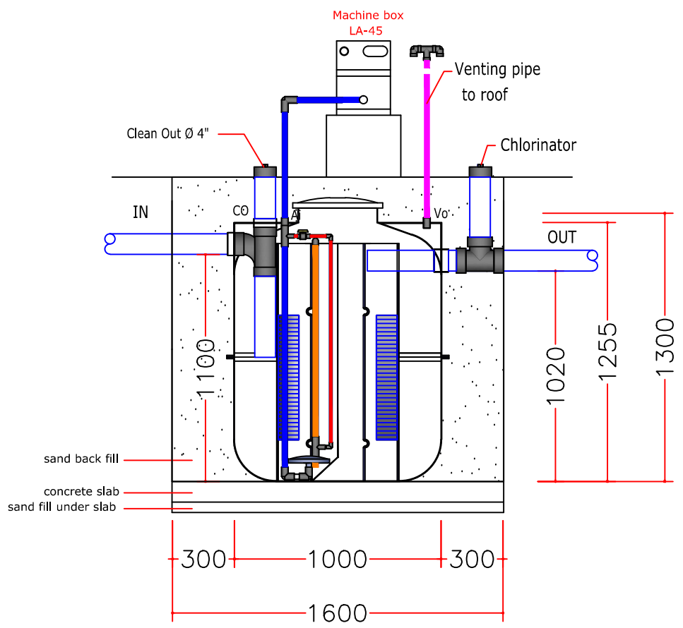
POTONGAN
