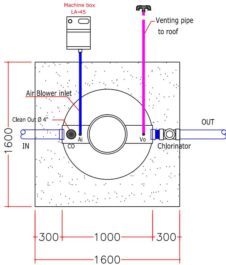
TAMPAK ATAS
