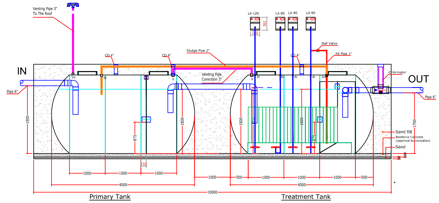
POTONGAN
