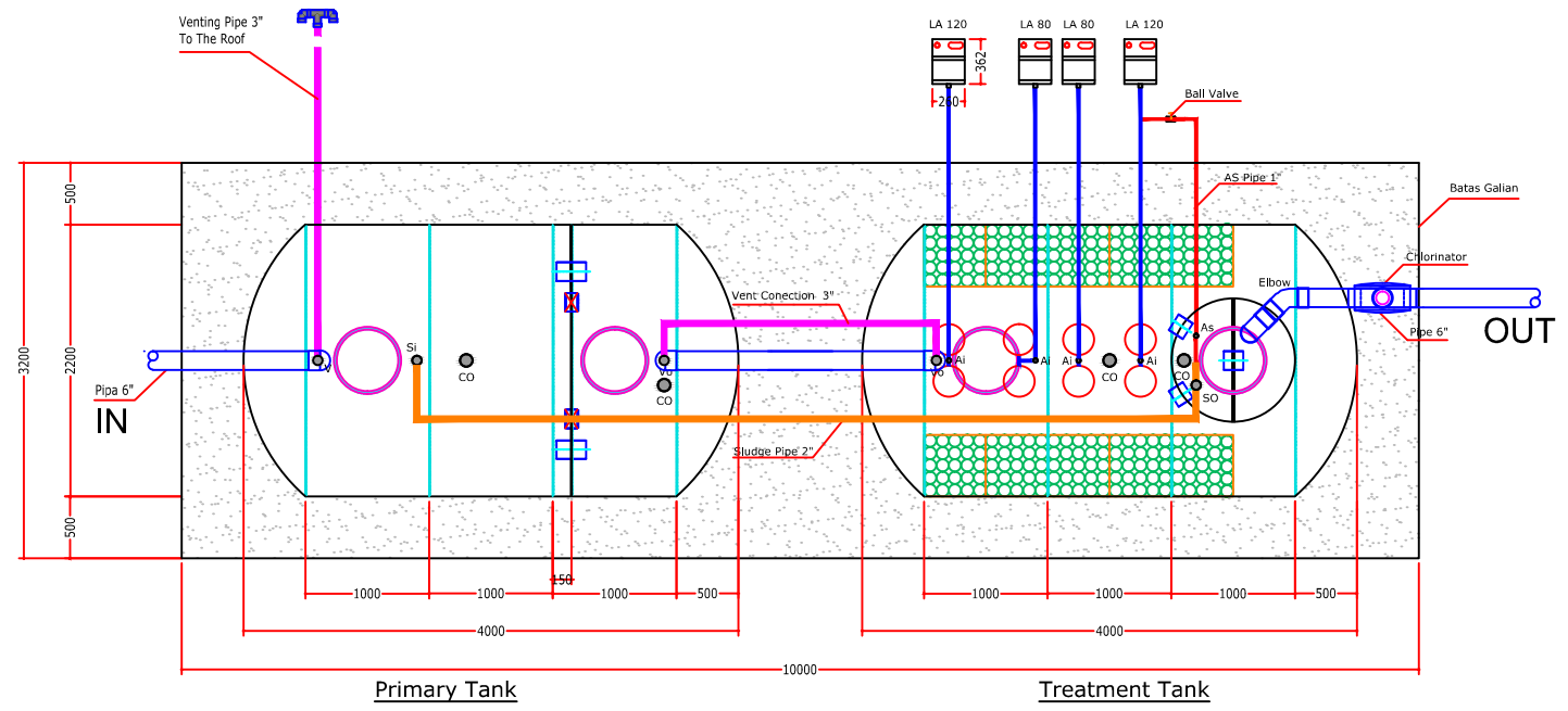
TAMPAK ATAS
