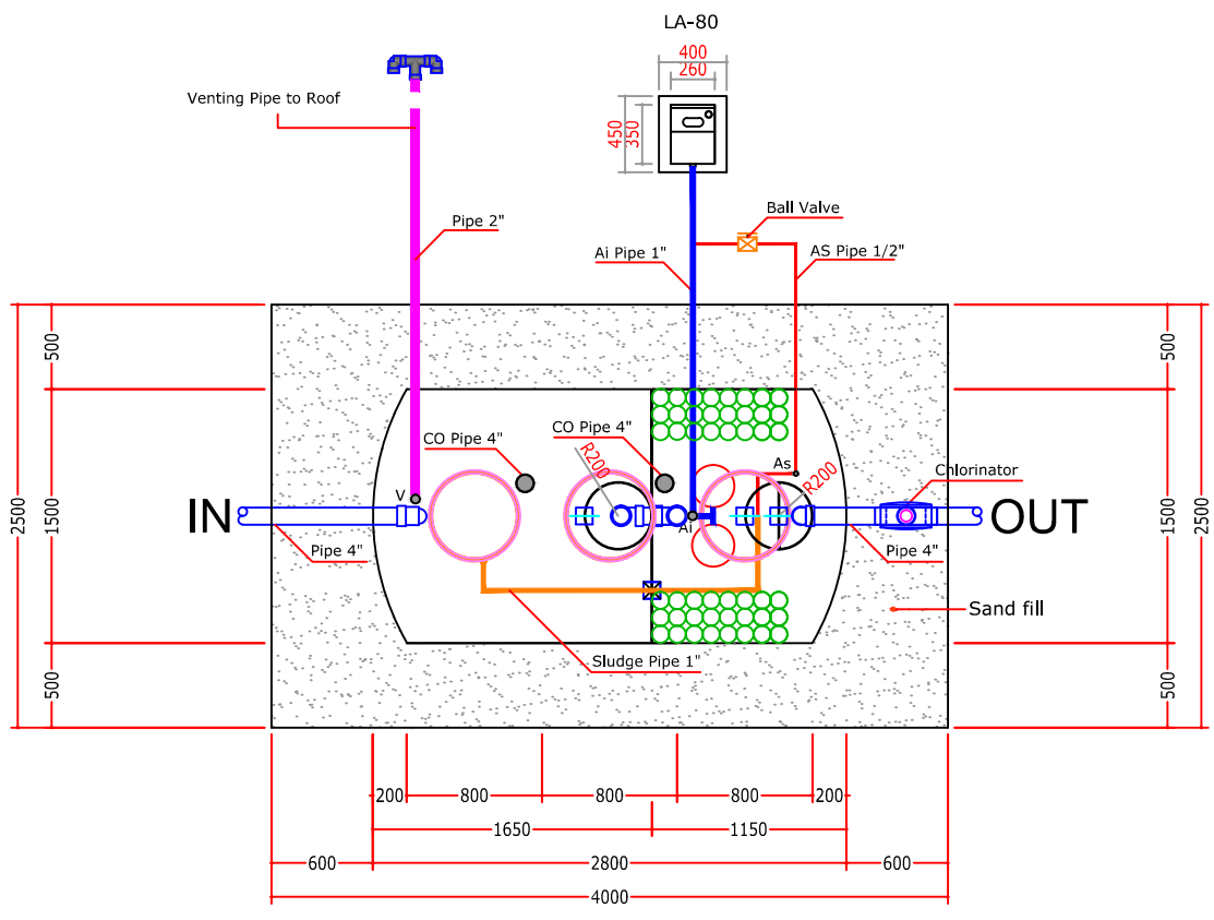
TAMPAK ATAS
